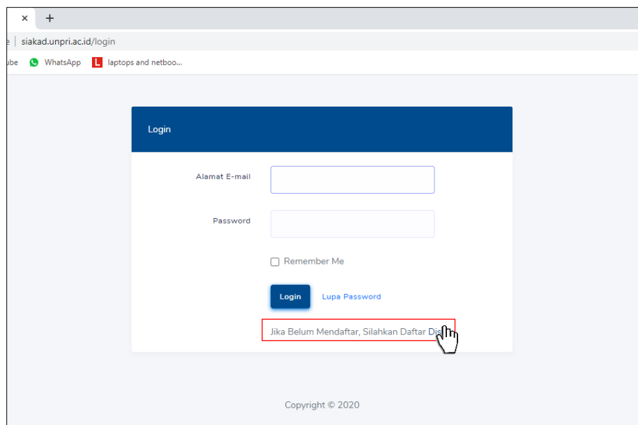
Gambar 2. Halaman login
