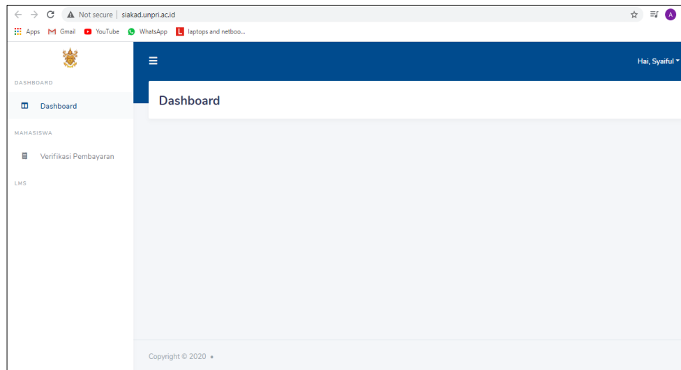
Gambar 7. Halaman mahasiswa
